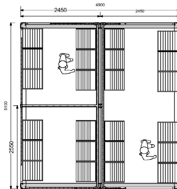
PIANTA PAVIMENTI
